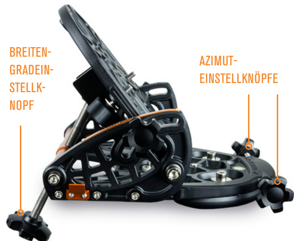
Abb. D4: Nehmen Sie Anpassungen am Keil mit den Azimut- und Breitengradeinstellknöpfen vor.
