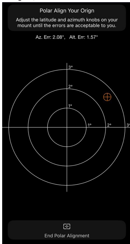
Abb. D3: Der Polausrichtungsbildschirm. Diese Grafik bietet eine visuelle Anleitung zur Einstellung des Äquatorialkeils. Der Azimutfehler wird auf der horizontalen Achse und der Höhenfehler auf der vertikalen Achse angezeigt. Wenn die Ausrichtung abgeschlossen ist, sollte das Fadenkreuz nahe der Mitte der Grafik liegen.
