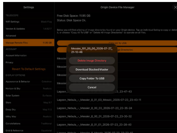
FIG I8: Téléchargez le Master empilé final pour chaque tuile sur un périphérique de stockage USB à partir de Menu > Paramètres > gérer les fichiers distants. Appuyez sur le dossier de la tuile, puis sélectionnez Copier le dossier sur USB. Si vous avez activé Enregistrer les images RAW, les fichiers au format RAW seront téléchargés aussi.
