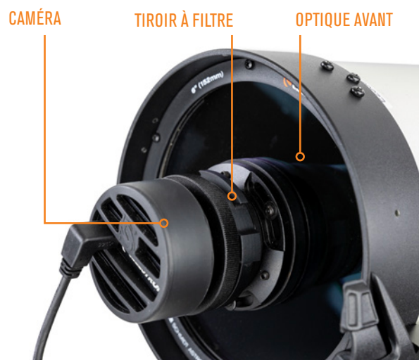
Fig. 14 Le tiroir à filtre est situé entre la caméra et l'optique avant.
