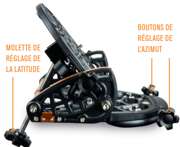
FIG D4: Réglez la cale à l'aide des boutons de réglage de l'azimut et de la latitude.
