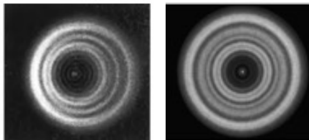
ABB. 33: Wenn die Optik ausgerichtet werden muss, ist das „Loch“ nicht in der Mitte des defokussierten Sternbilds.
