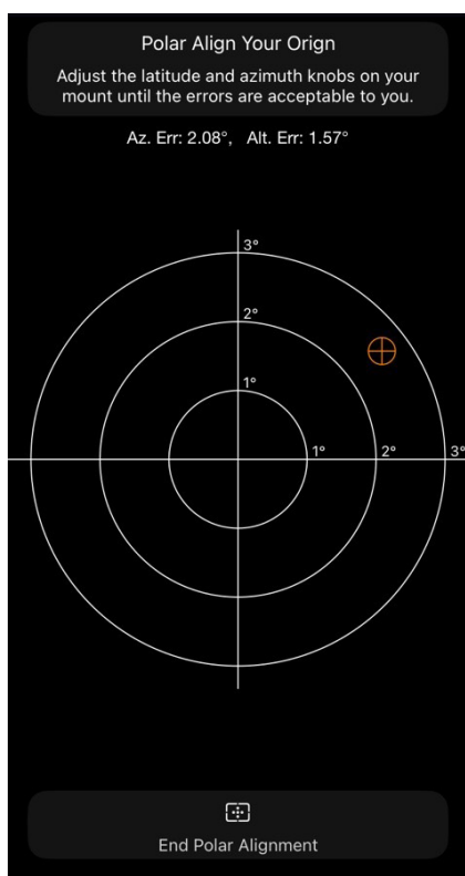
FIG D3: schermata di Allineamento Polare. Questo grafico fornisce una guida visiva per la regolazione del cuneo. L'errore di azimuth è mostrato sull'asse orizzontale e l'errore di altitudine sull'asse verticale. Una volta completato l'allineamento, l'indicatore a croce dovrebbe trovarsi vicino al centro del grafico.
