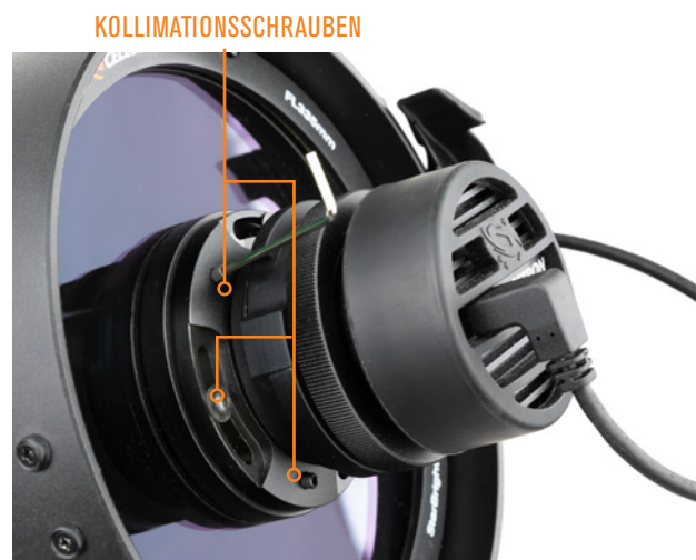
ABB. 34: Justieren Sie die Neigung der Linsengruppe (und der Kamera) mit den Kollimationsschrauben.
