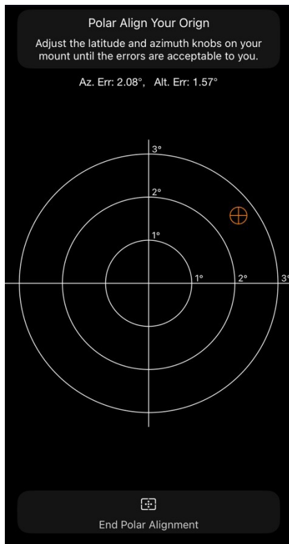
FIG D3: Écran d'alignement polaire. Ce graphique fournit un guide visuel pour le réglage de la cale. L'erreur d'azimut est indiquée sur l'axe horizontal et l'erreur d'altitude sur l'axe vertical. Une fois l'alignement terminé, le réticule doit être proche du centre du graphique.
