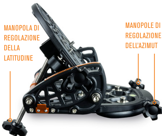
FIG D4: Regolare il cuneo utilizzando le manopole di regolazione dell'azimut e della latitudine.
