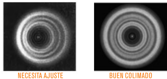
FIG 33: Si la óptica precisa de alineación, el "agujero" no estará centrado en la estrella desenfocada.
