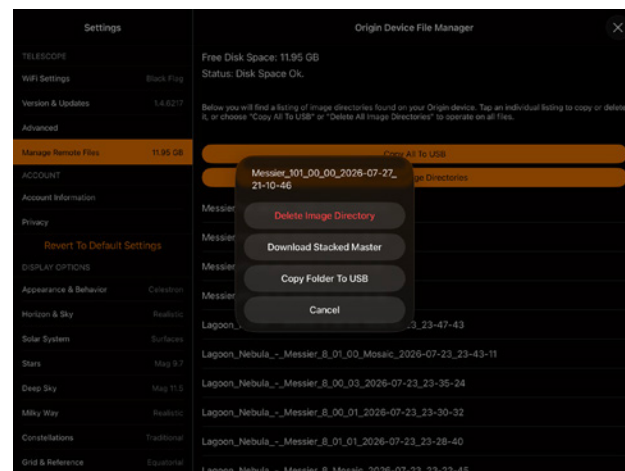
FIG I8: Descargue el maestro apilado final para cada lámina en una unidad USB desde Menú > Configuración > Gestionar archivos remotos. Toque la carpeta del archivo y seleccione Copiar carpeta a USB. Si ha activado Guardar imágenes RAW, los archivos de imagen RAW también se descargarán.
