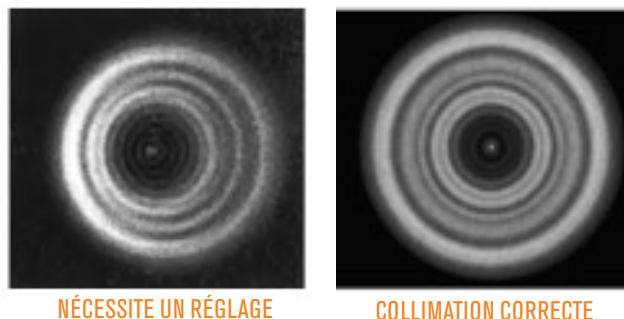
Fig 33 Si l'optique a besoin d'être alignée, le "trou" ne sera pas centré dans l'image de l'étoile défocalisée.
