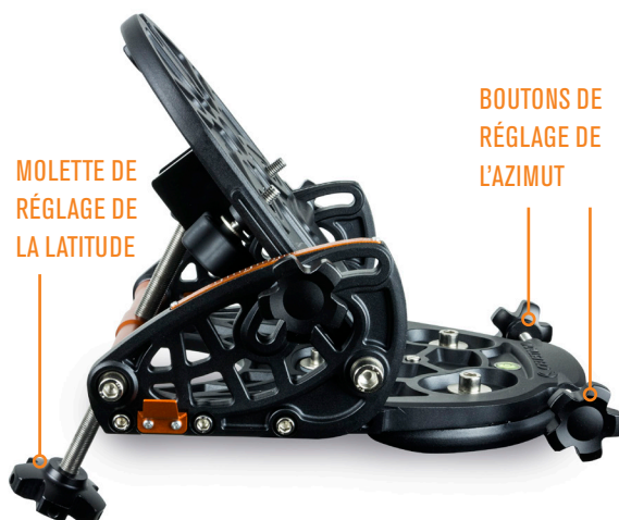
FIG D4: Réglez la cale à l'aide des boutons de réglage de l'azimut et de la latitude.
