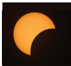
ÉCLIPSE PARTIELLE
