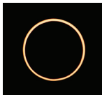
ÉCLIPSE ANNULAIRE
